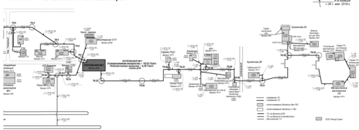
Рисунок 29 Схема теплоснабжения объектов от котельной ПЧ Забайкальской дирекции по тепловодоснабжению (часть 2)
