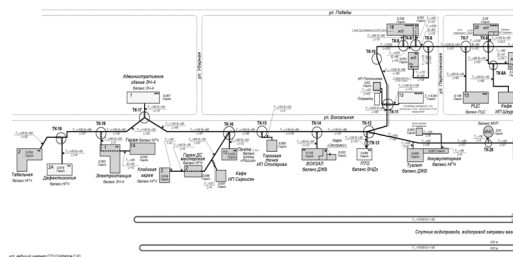
Рисунок 27 Схема теплоснабжения объектов от котельной ВОХР Забайкальской дирекции по тепловодоснабжению
