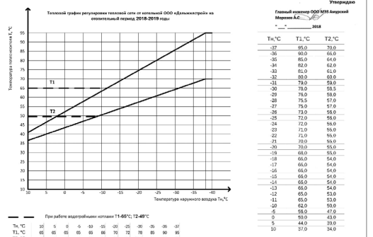
Рисунок 25 Температурный график сетевой воды, отпускаемой котельной ООО "Дальжилстрой"
