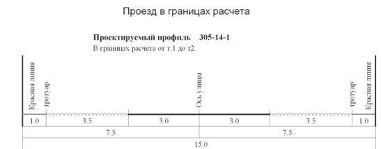
Разбивочный чертеж красных линий
