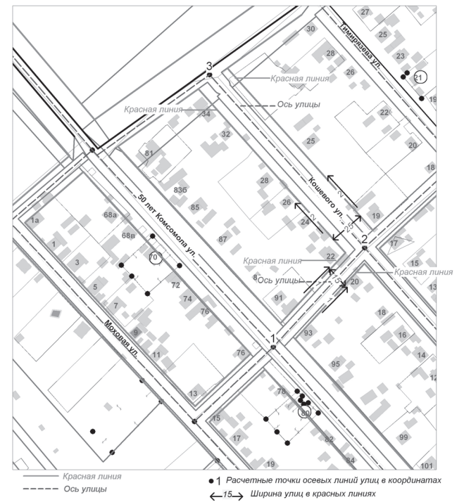
Разбивочный чертеж красных линий в квартале № 256
